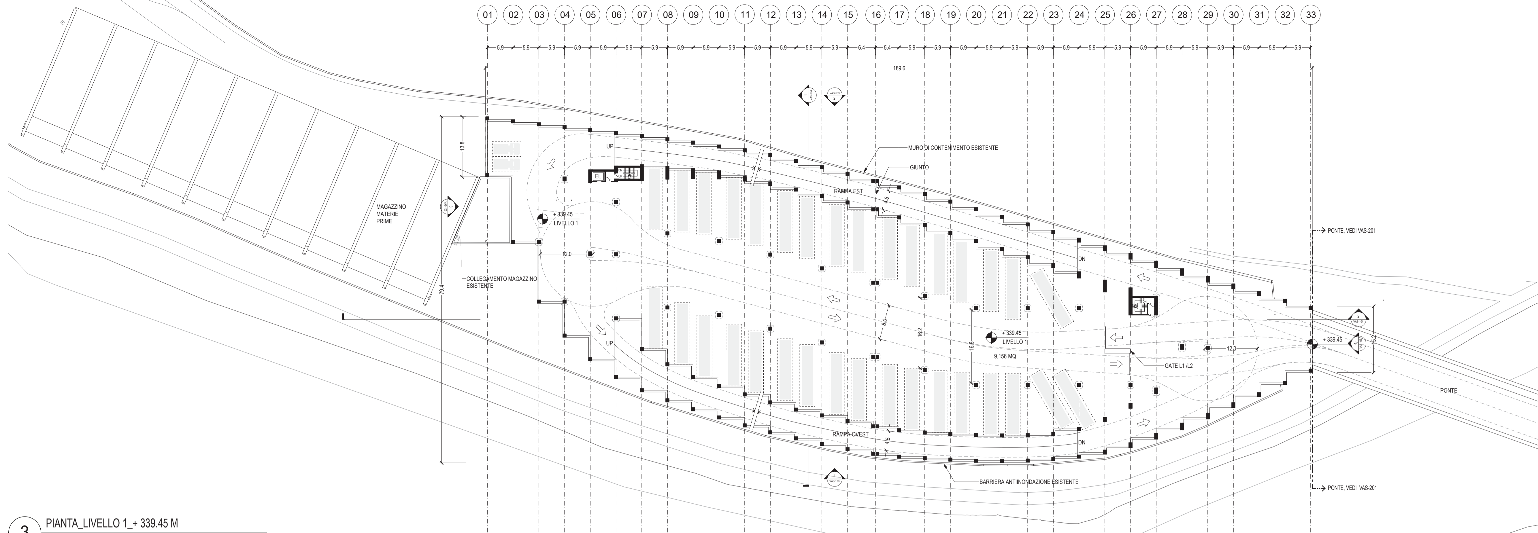
3 PIANTA LIVELLO 1_+ 339.45 M
