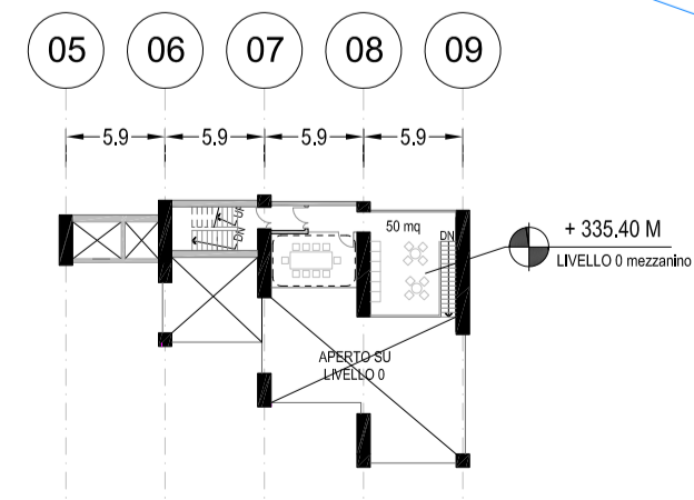
2 UFFICI - LIVELLO MEZZANINO_+335.40 M
